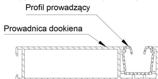
Rys. 5. Prowadnica dookienna - elementy
