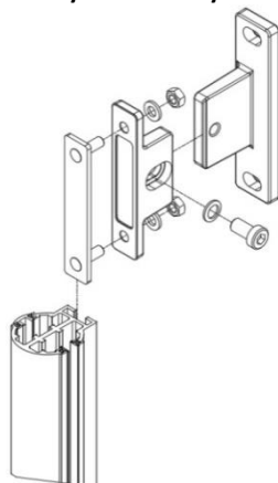
Prowadnica OVAL (okrągła)
