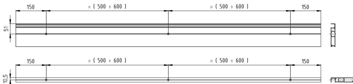
Rys. 14. Schemat wykonywania otworów montażowych w profilu prowadnicy.
