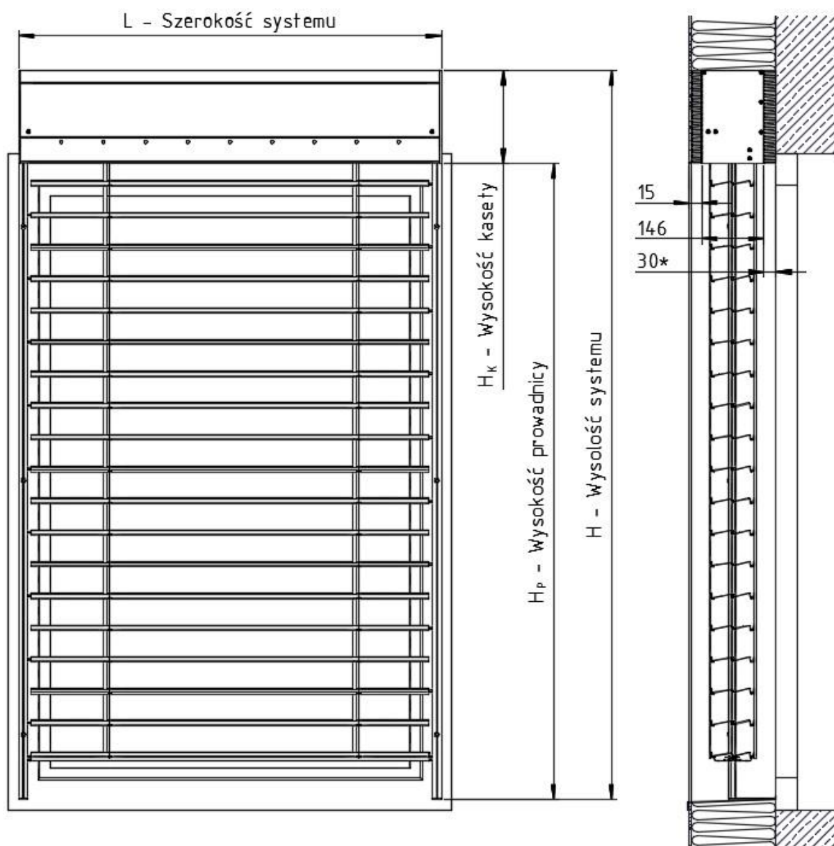
Rys. 11. Wymiary systemu żaluzji fasadowych Z90 z kasetą podtylnkową. * - Wymiar zmienny, standardowo 30 mm.
