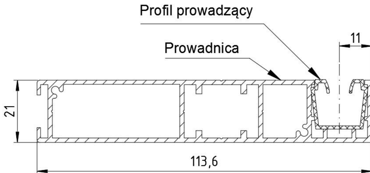
Rys. 9. Prowadnicą do systemu z kasetą podtynkową – elementy.
