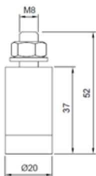
Napinacz fasadowy
