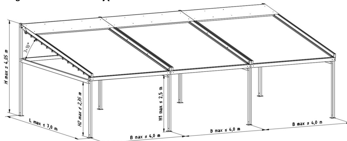
Rys. 2. Pergola Solid wolnostojąca wielomodułowa - Wymiary gabarytowe: B max – szerokość maksymalna modułu, L max – długość maksymalna (standard 3,85 m), H max – wysokość maksymalna, H1 max – prześwit w świetle belki przedniej (standard 2,30 m), H2 max – prześwit w świetle belki bocznej i tylnej (standard 2,15 m).
