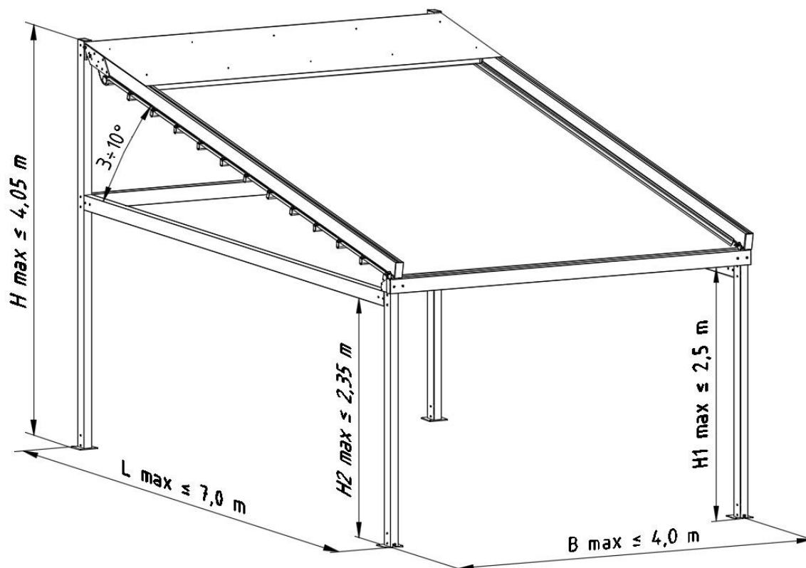
Rys. 1. Pergola Solid wolnostojąca jednomodułowa - Wymiary gabarytowe: B max – szerokość maksymalna modułu, L max – długość maksymalna (standard 3,85 m), H max – wysokość maksymalna, H1 max – prześwit w świetle belki przedniej (standard 2,30 m), H2 max – prześwit w świetle belki bocznej i tylnej (standard 2,15 m).
