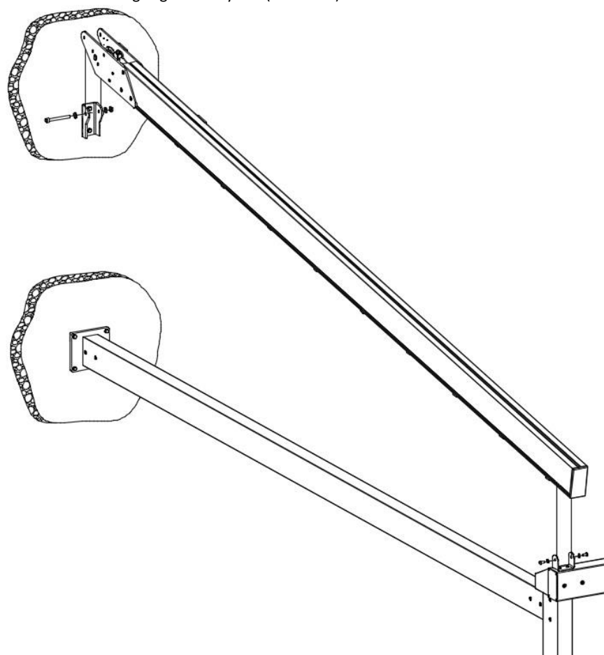
Rys. 41. Sposób montażu Belki prowadzącej.
