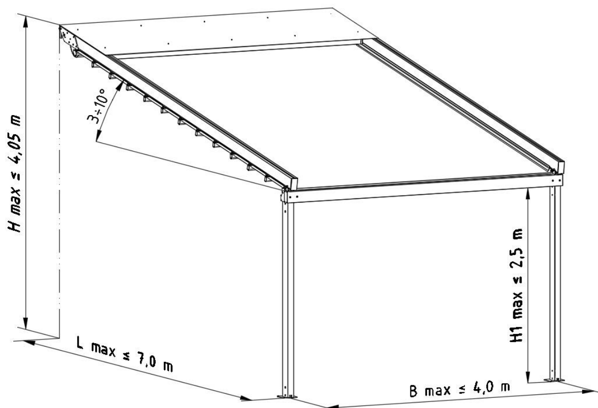
Rys. 3. Pergola Solid przyścienna jednomodułowa - Wymiary gabarytowe: B max – szerokość maksymalna modułu, L max – długość maksymalna (standard 3,85 m), H max – wysokość maksymalna, H1 max – prześwit w świetle belki przedniej (standard 2,30 m).
