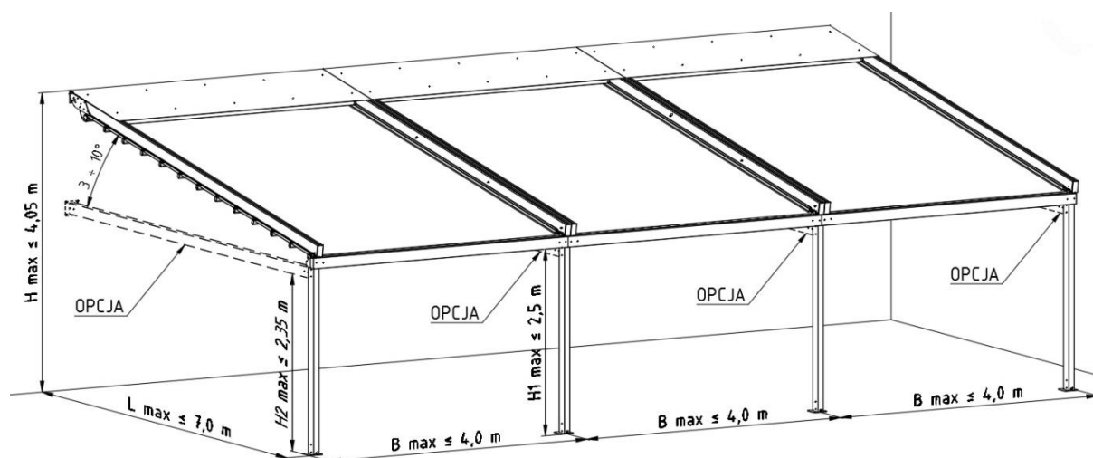
Rys. 4. Pergola Solid przyścienna wielomodułowa - Wymiary gabarytowe: B max – szerokość maksymalna modułu, L max – długość maksymalna (standard 3,85 m), H max – wysokość maksymalna, H1 max – prześwit w świetle belki przedniej (standard 2,30 m), H2 max – prześwit w świetle belki bocznej i tylnej (standard 2,15 m).
